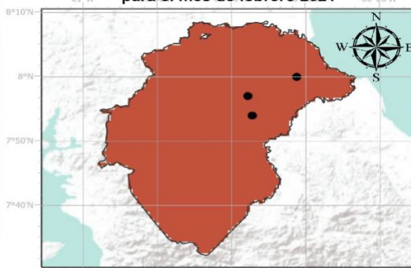
Valores esperados de lluvia en milímetros (mm) para el mes de febrero 2021
